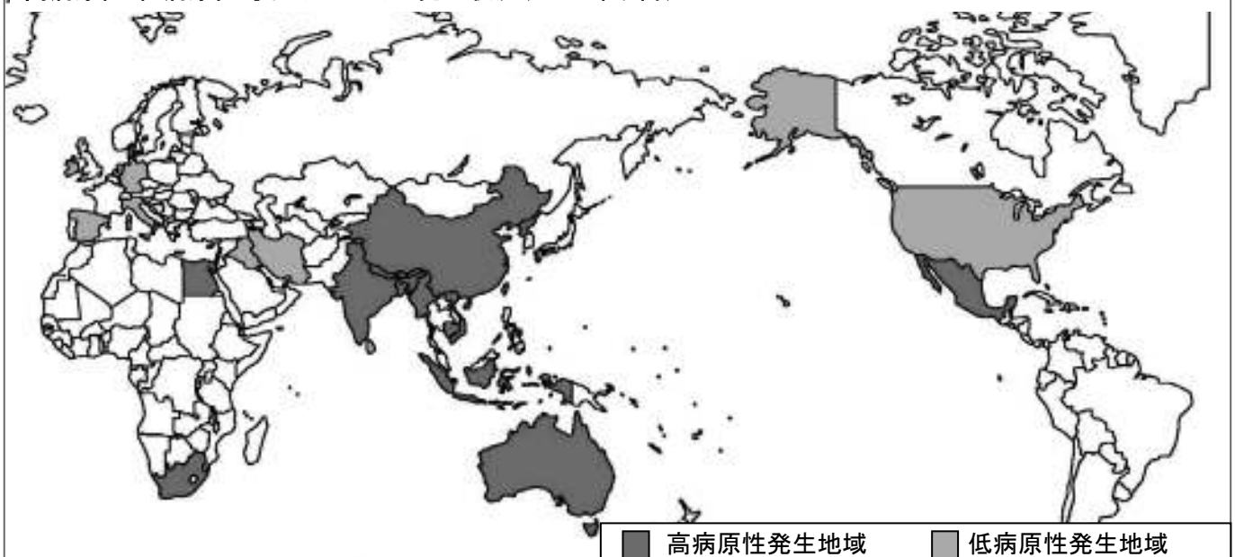
高病原性・低病原性鳥インフルエンザの発生状況 (2012 年以降)
